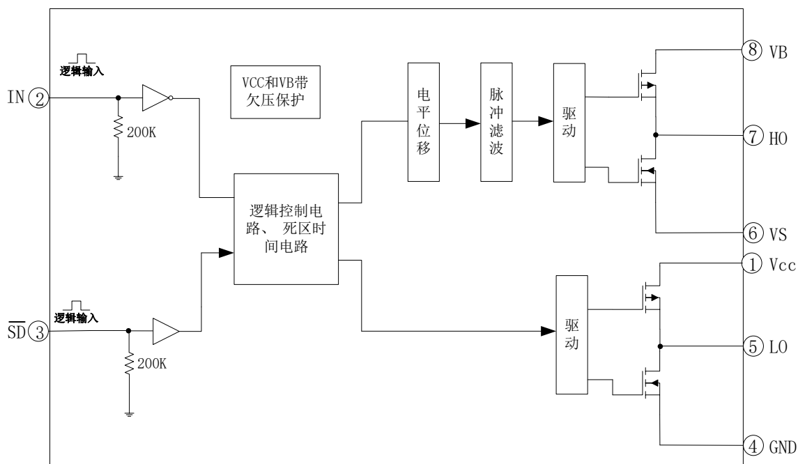
图 5-1. EG2104M 内部电路图
