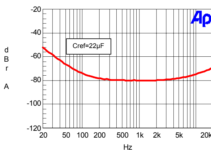
PSRR
