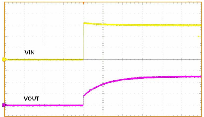
VIN : 1.0V/div, VOUT : 1.0V/div, Time : 50ms/div
