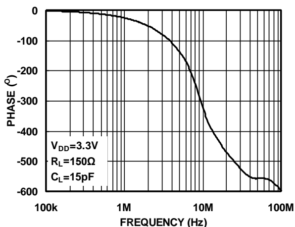
图5. 相位与频率的关系
