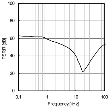
Fig.19 PSRR (Io=0mA)
