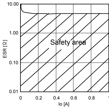
Fig.17 ESR Condenser
