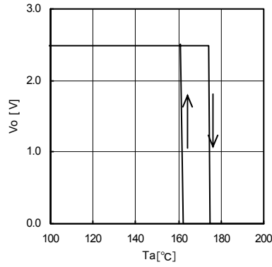
Fig.14 TSD (Io=0mA)
