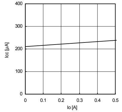
Fig.18 Io-Icc
