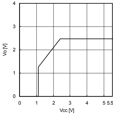
Fig.13 Vcc-Vo (Io=0mA)
