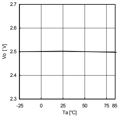
Fig.7 T_a - V_o ( I_o=0\text{mA} )
