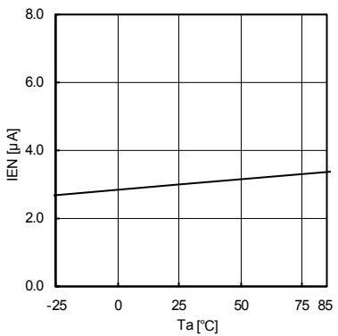
Fig.10 T_a - I_{EN}
