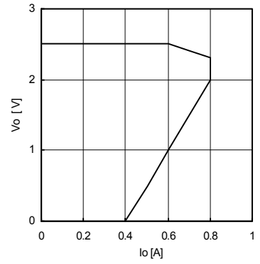
Fig.15 OCP
